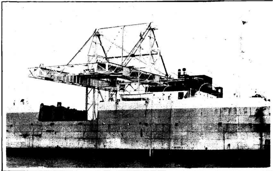
Esta grúa "Shaw", que alza su estructura formidable sobre el puente del "Seatrain", es capaz de levantar un peso de 105 toneladas. Sus poderosos cables suspenden los vagones cargados y los colocan con suavidad en la cala del buque.
