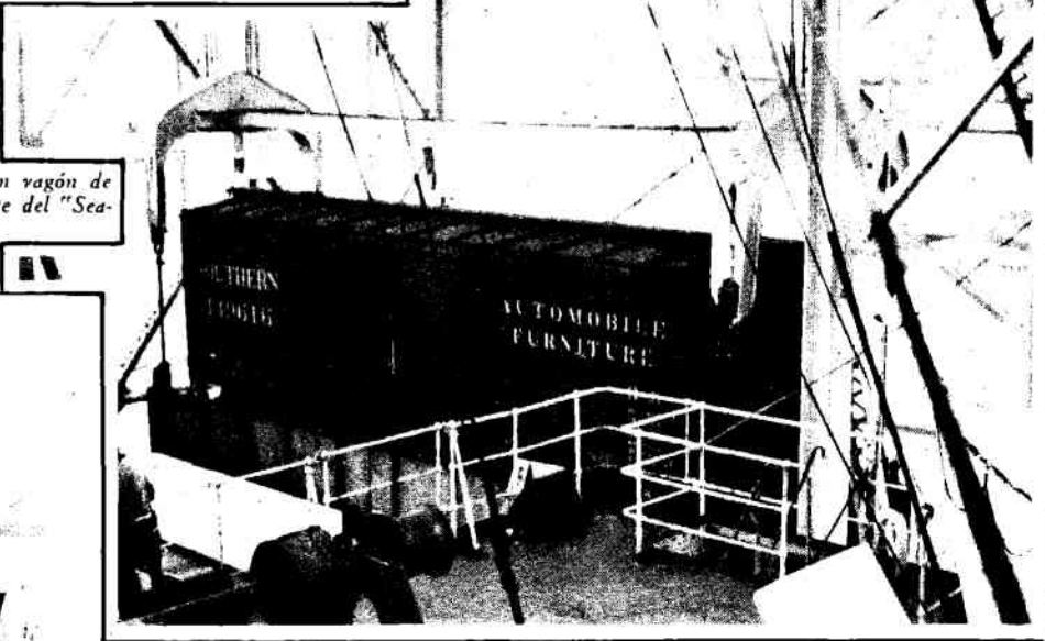
Esta grúa "Shaw", que alza su estructura formidable sobre el puente del "Seatrain", es capaz de levantar un peso de 105 toneladas. Sus poderosos cables suspenden los vagones cargados y los colocan con suavidad en la cala del buque.
